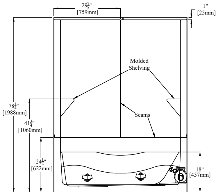
ELEVATION
